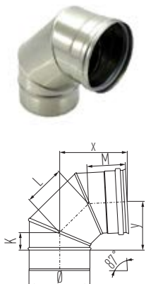
Elbow 87°
