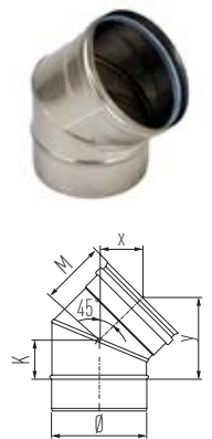
Elbow 45°
